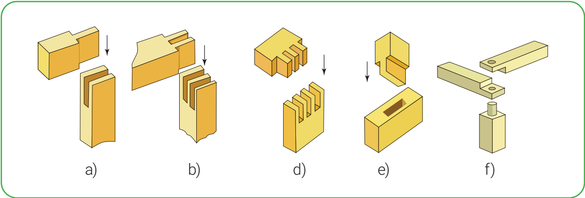
21-rasm. Duradgorlik birikmalarini bog'lash usullari: a) bir tirnoqli; b) ikki tirnoqli; d) uch tirnoqli; e) to'g'ridan to'g'ri yopiq tirnoqli; f) zakrovli birikma.
