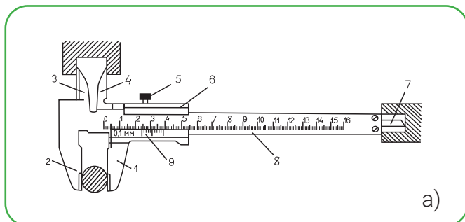
24-rasm. SHTS-1 markali shtangensirkul: a) tuzilishi: 1, 4 – qoʻzgʻaluvchan jagʻlari; 2, 3 – qoʻzgʻalmas jagʻlar; 5 – qotiruvchi vint; 6 – hisob olish; 7 – glubinomer (chuqurlikni oʻlchaydigan sterjen); 8 – shtanga; 9 – nonius; b) hisob olish.
