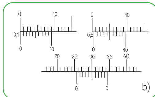
24-rasm. SHTS-1 markali shtangensirkul: a) tuzilishi: 1, 4 – qoʻzgʻaluvchan jagʻlari; 2, 3 – qoʻzgʻalmas jagʻlar; 5 – qotiruvchi vint; 6 – hisob olish; 7 – glubinomer (chuqurlikni oʻlchaydigan sterjen); 8 – shtanga; 9 – nonius; b) hisob olish.
