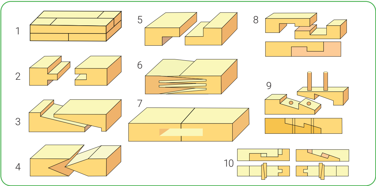
22-rasm. Duradgorlikda qo'llaniladigan ulab uzaytirish usullari: 1 – uchma-uch; 2 – taroqli; 3 – suyri usulda; 4 – ponasimon; 5 – kertmakli; 6 – ponasimon; 7 – qistirma ponali; 8 – ustma-ust qulf usulida; 9 – pog'onali mix cho'pli usulda; 10 – taranglanadigan to'g'ri qulf va qiya usulda.
