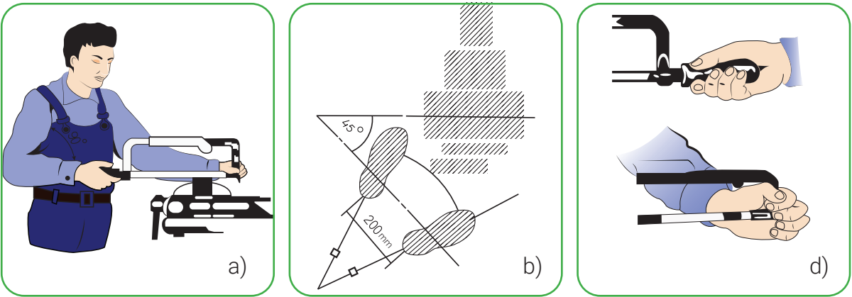
34-rasm. Arralash vaqtida to'g'ri ish vaziyatini tanlash: a) ish o'rnining balandligini aniqlash; b) ish o'rniga nisbatan turish; d) arrani tutish.
