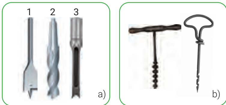
15-rasm. Parmalar: a) parma turlari: 1 – perosimon, 2 – spiralsimon, 3 – novsimon; b) qo'l parm alari.
