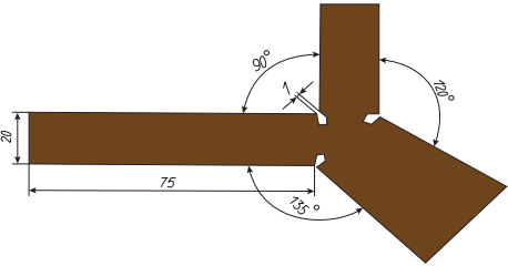
29-rasm. Kombinatsiyalashgan goʻniya.
